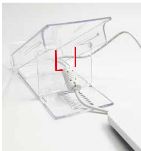
③CIR315A のコードを開口にフェライト（円柱のボックス）を通します
